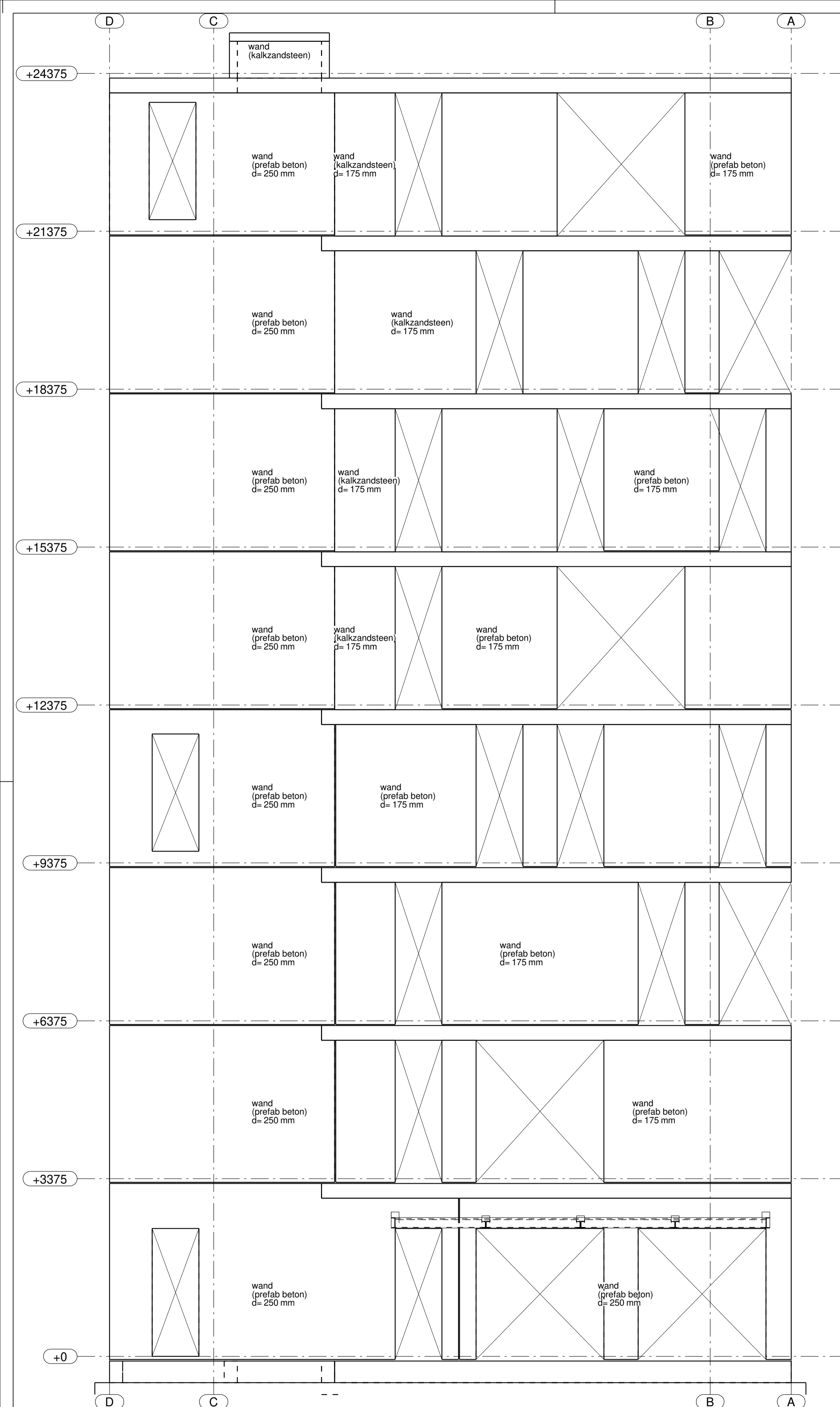
Gevelaanzicht as 01 1:50
