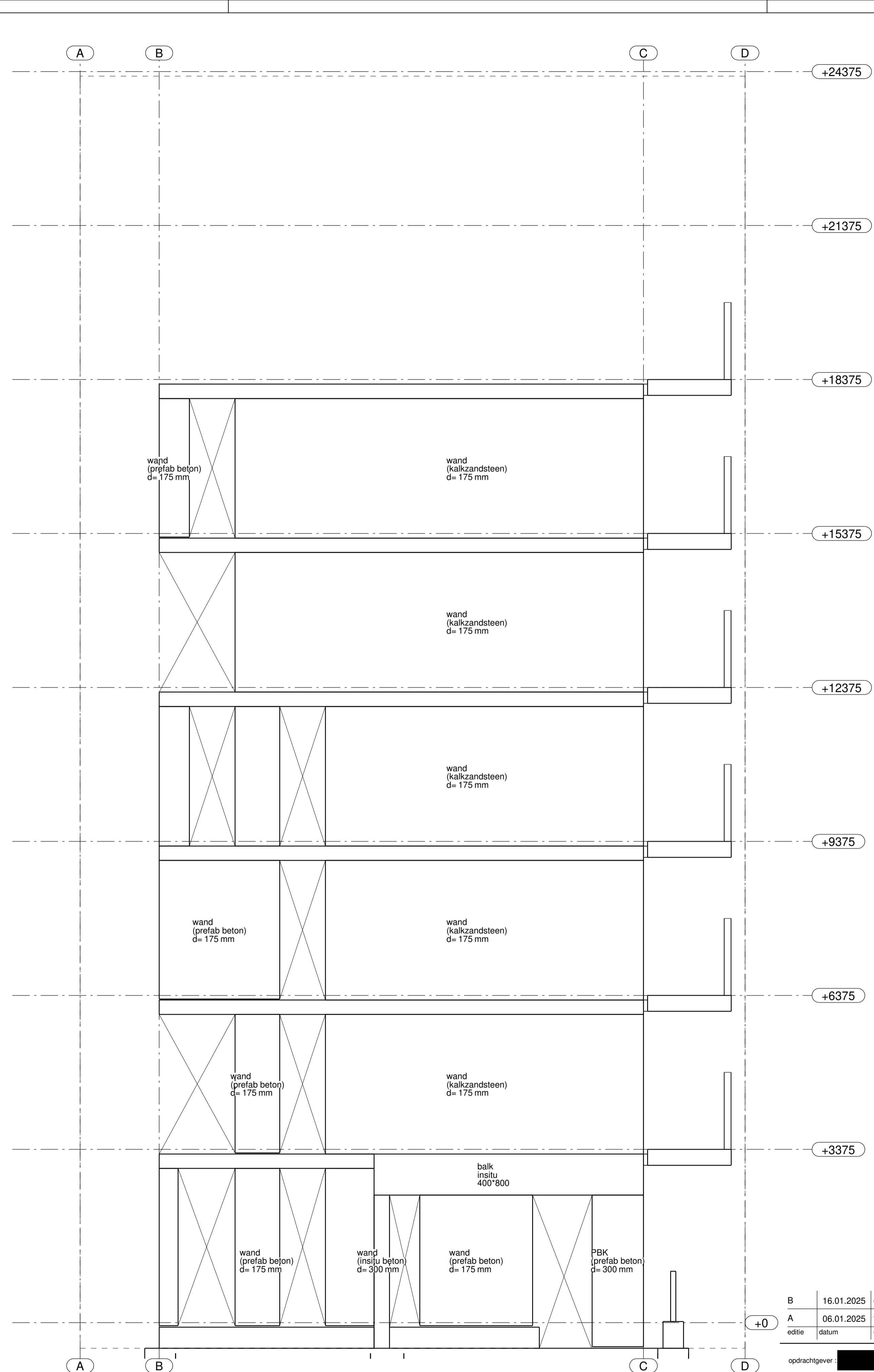
Gevelaanzicht as 05 1:50
