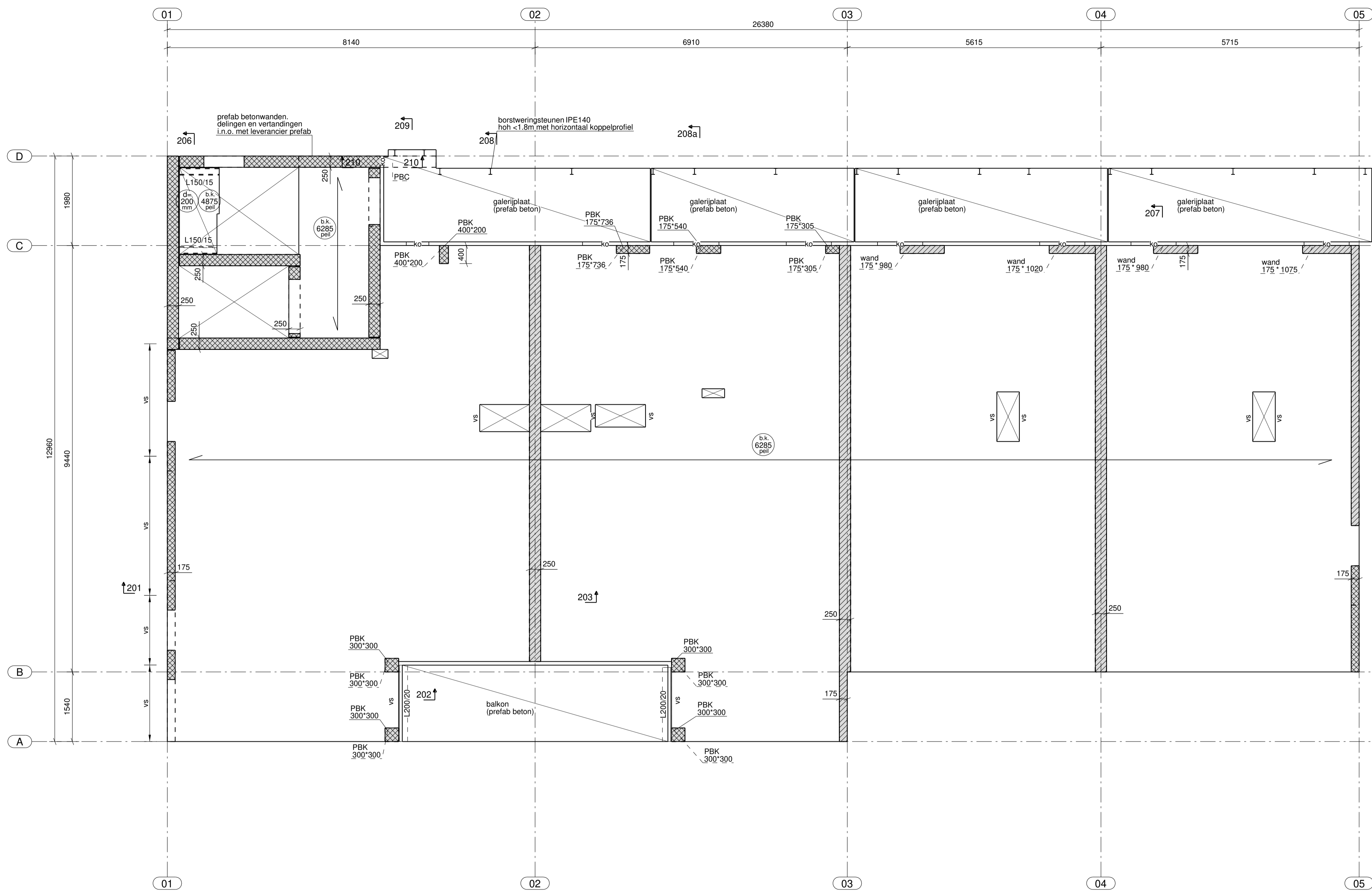
Tweede verdiepingsvloer 1:50
