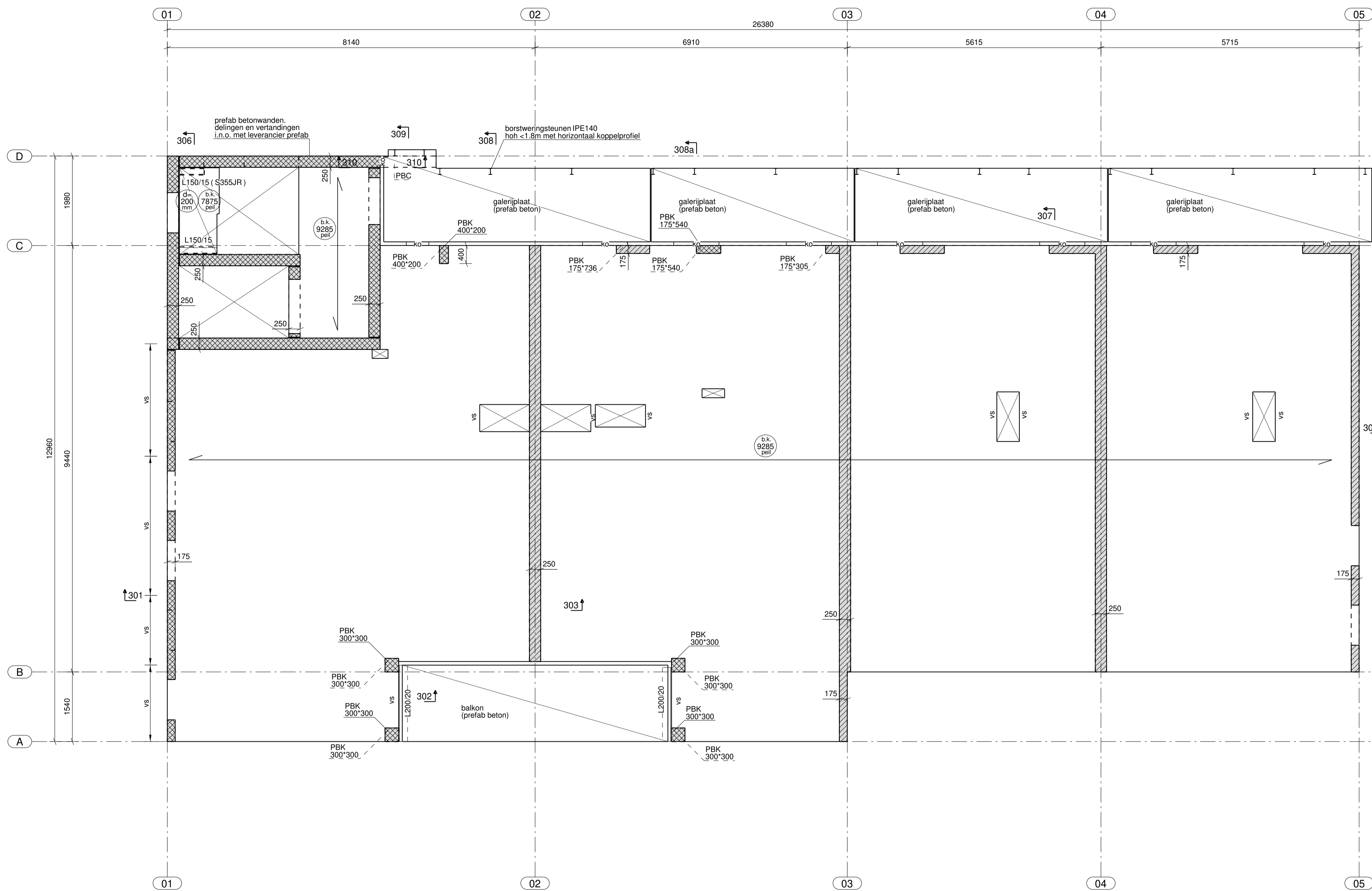
Derde verdiepingsvloer 1:50
